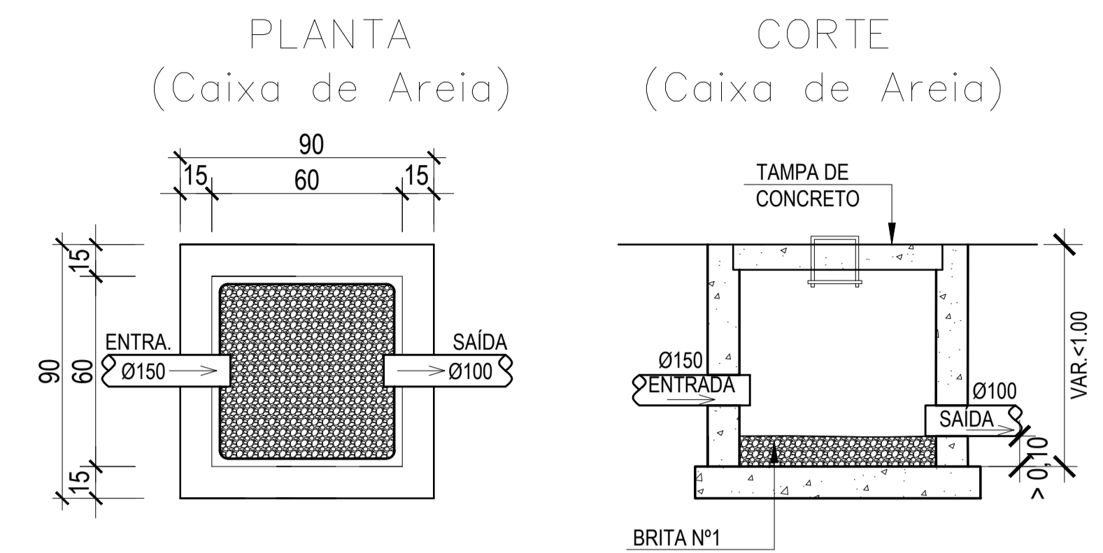
DETALHE CAIXA DE AREIA SEM ESCALA
