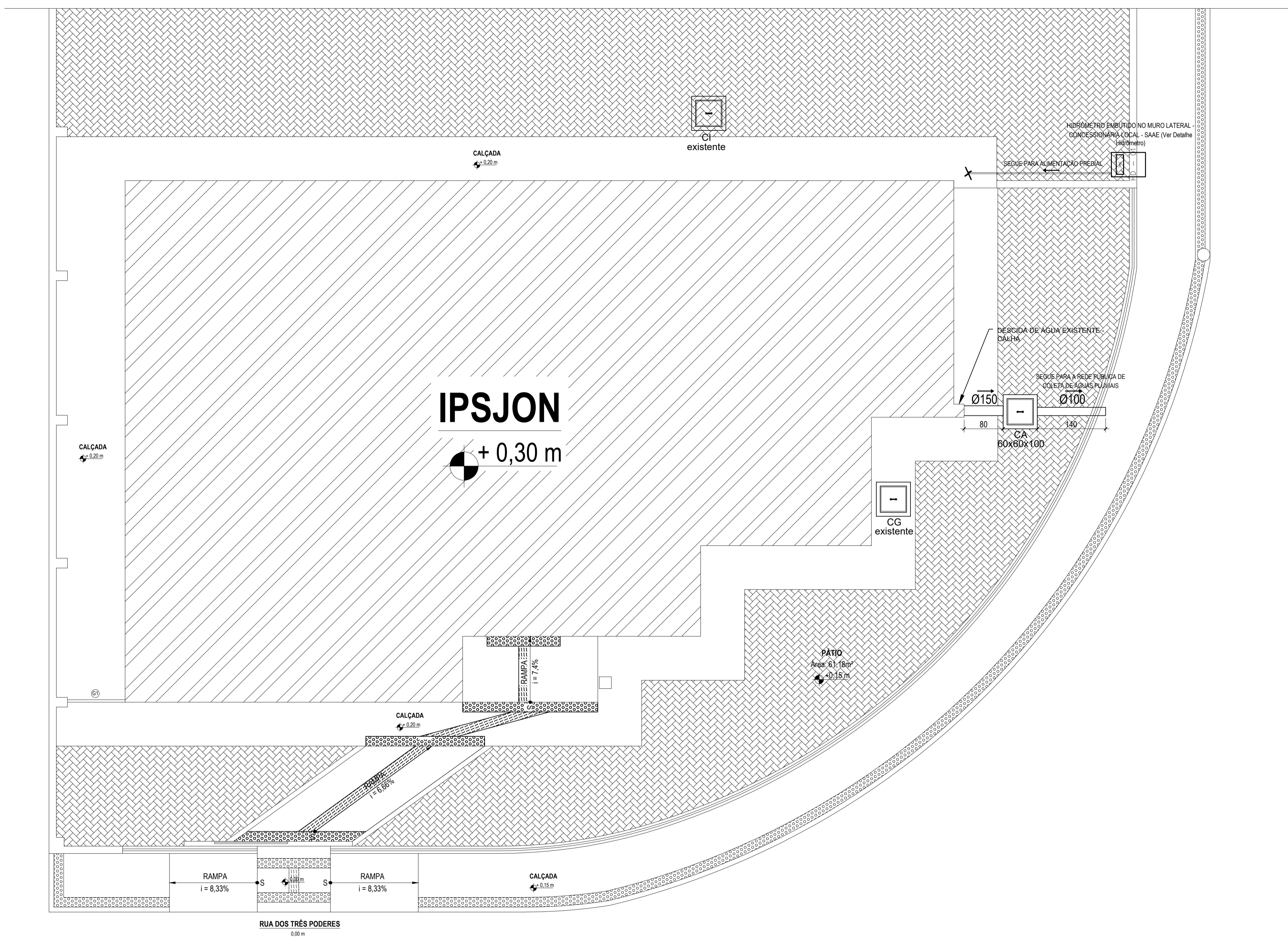
ESQUEMA HORIZONTAL ESGOTO ESCALA: 1/50
